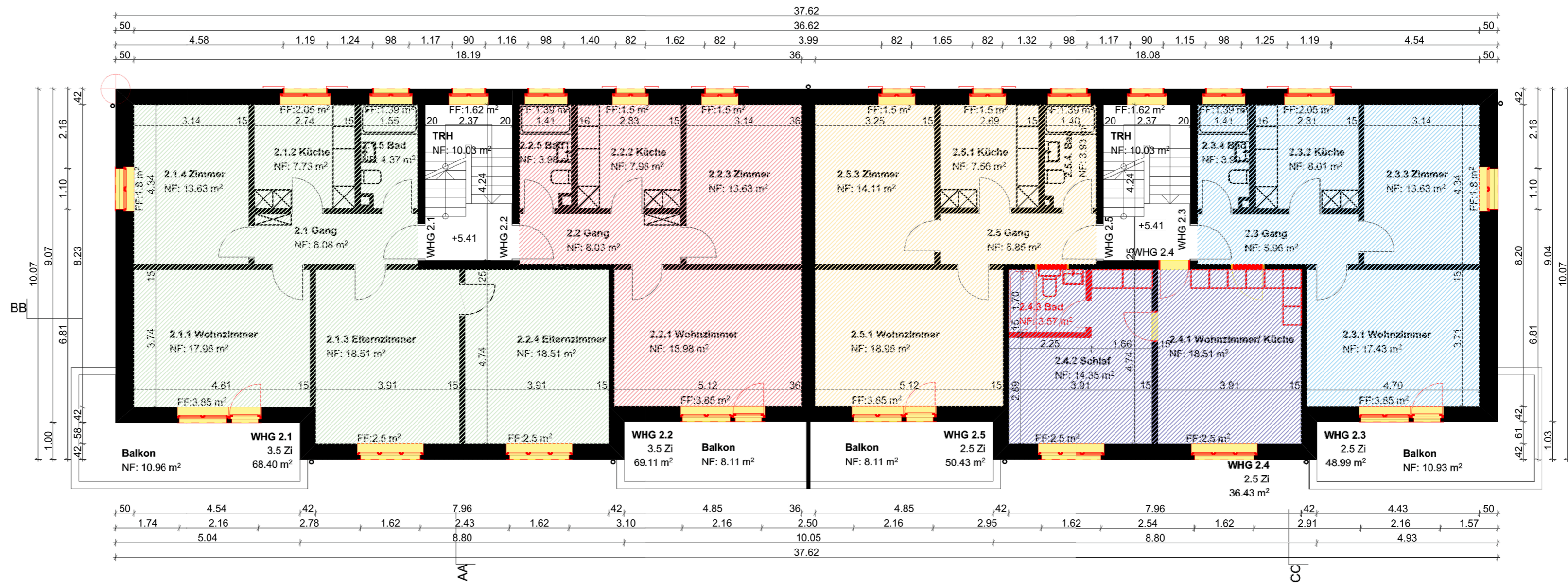
Obergeschoss 2
